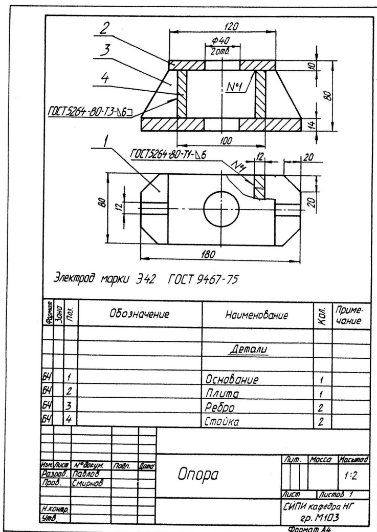
Рис. 17. Пример выполнения задания по теме «Соединения сварные»
