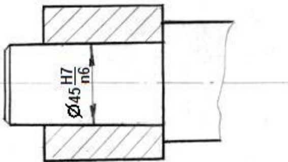
эскиз узла с заданной посадкой и деталей узла
