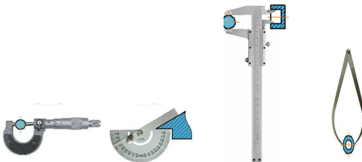
Рис. 6 Измерительные инструменты сварщика
